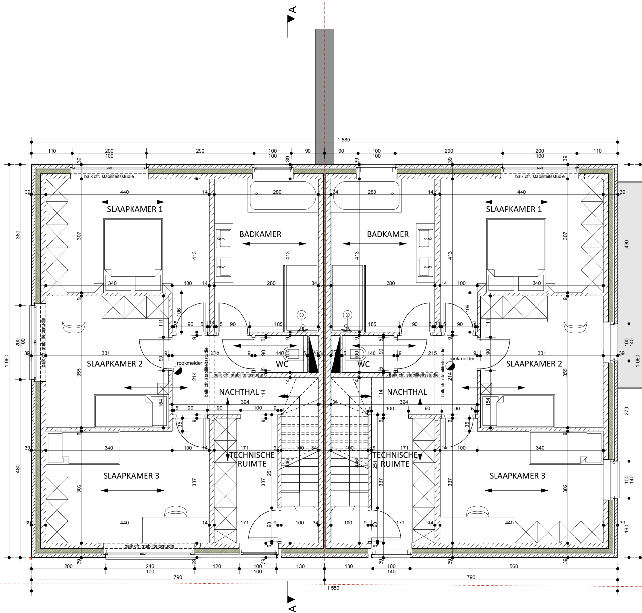
VERDIEPING 1 WONINGEN BLOK A
